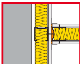
Rys. 5: Zalecane rozwiązania montażowe ścian działowych dla zmniejszenia bocznego przenoszenia dźwięków.
