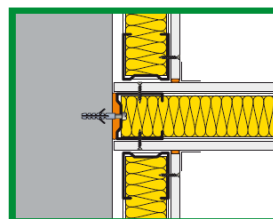
Rys. 5: Zalecane rozwiązania montażowe ścian działowych dla zmniejszenia bocznego przenoszenia dźwięków.
