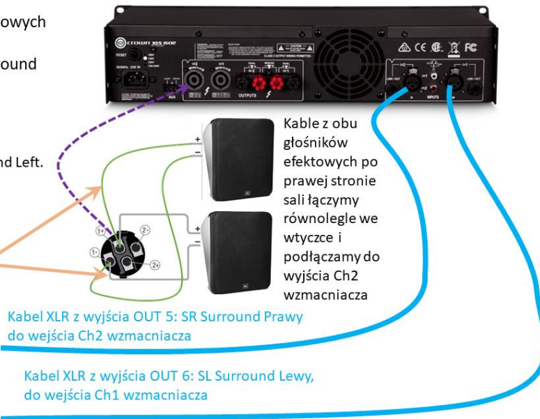
Rys. 70: Podłączenie kolumn efektowych po prawej stronie sali.
