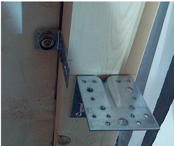
Rys. 29: Zawiesie mocujące słupek do ściany konstrukcyjnej za pomocą wkrętu z podkładką i łącznik przygotowany do przykręcenia belki poziomej. Między belką a ścianą widoczna czarna mata izolacyjna IZOPLAST PREMIUM 10 mm.
