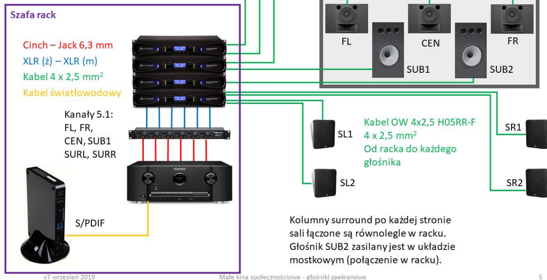
Rys. 65: Schemat połączeń systemu nagłośnienia.
